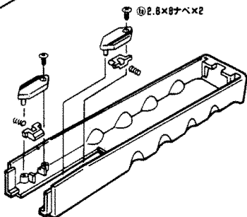
SV-8 SUPER VERSION フォアグリップ
